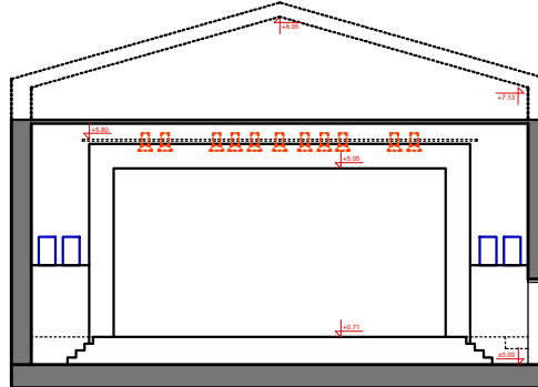
POPRECNI PRESEK - POGLED KA BINI
