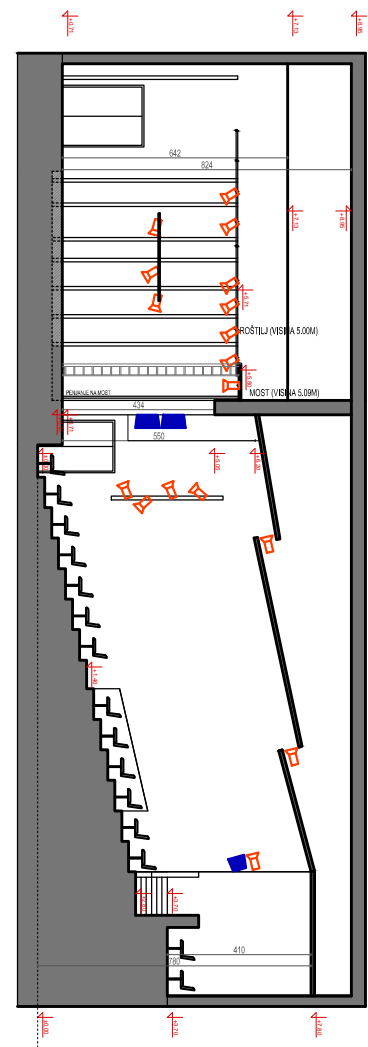
PODUZNI PRESEK
